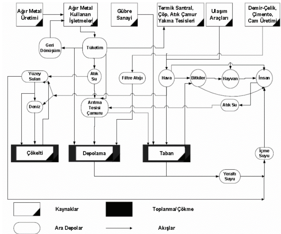
Şekil 1. Şematik olarak ağır metallerin doğaya yayınımları (Duffus ve Worth, 1996)
