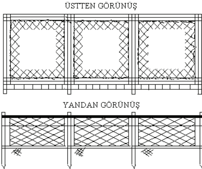
Şekil 10. Sabit kafesler (Atay, 1987)
