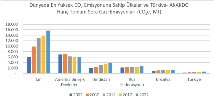
Şekil 2. Dünyada En Yüksek CO 2 Emisyonuna Sahip Ülkeler ve Türkiye- AKAKDO Hariç Toplam Sera Gazı Emisyonları (CO 2 eşdeğeri, Mt)
