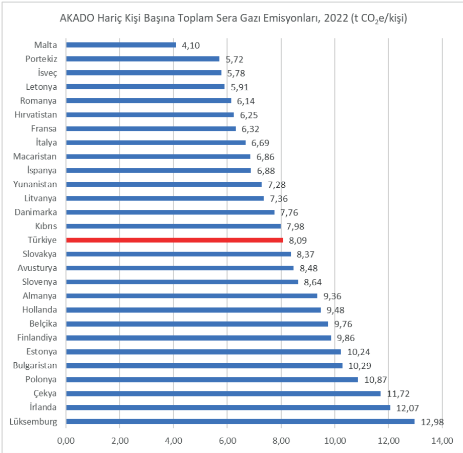
Şekil 5. AB27 Ülkeleri ve Türkiye'nin Kişi Başına Toplam Sera Gazı Emisyonları (ton/kişi)
