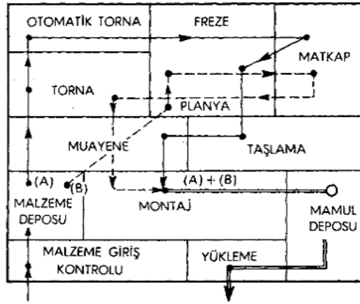
Şekil 5: Prosese göre yerleşim tipi
