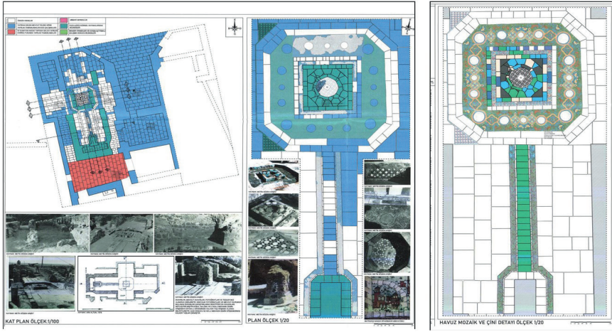
Artuklu Sarayı Röleve ve Restitüsyon Planları-2022.
