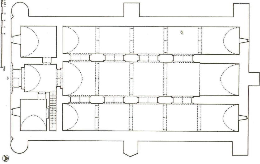
Çizim: 4- Bitlis Bapşin Hanı 'nın Planı (S. Erken'den).
