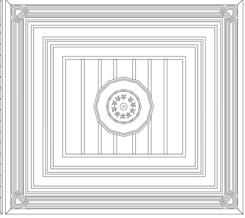
Őekil 2. 1 numaralı ev tavan çizimi
