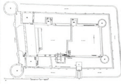
Çiz. 4: Çeşme Kalesi Plan (İ.A.Yüksel'den)
