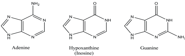
Şekil 2. Pürin bazlarının yapısı. Hipoksantin inozinin nükleobazıdır (Burgis, 2016).
