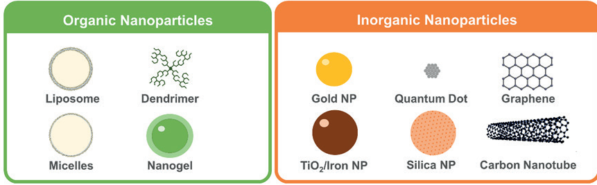
Şekil 1: Nanopartiküllerin sınıflandırılması. Nanopartiküller iki grupta sınıflandırılabilir: organik (lipidler, proteinler veya polimerler) ve inorganik (metaller veya tuzlar).
