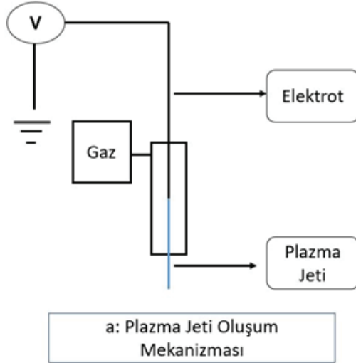
Şekil 1: Plazma jeti oluşum mekanizması
