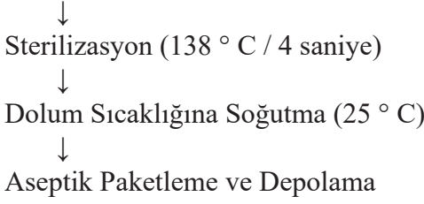
Şekil 6.2. a) Salep içeceğinde kullanılan sütün hazırlanışının akış diyagramı b) UHT işlemi uygulanmış salep içeceğinin hazırlık akış diyagramı.
