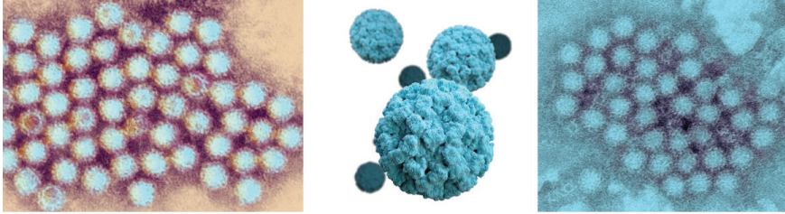
Şekil 1. Norovirüsün Elektron Mikroskobu ile Görünümü ( https://www.alamy.com/stock-photo/norovirus-micrograph.html?imgt=0&sortBy=relevant )
