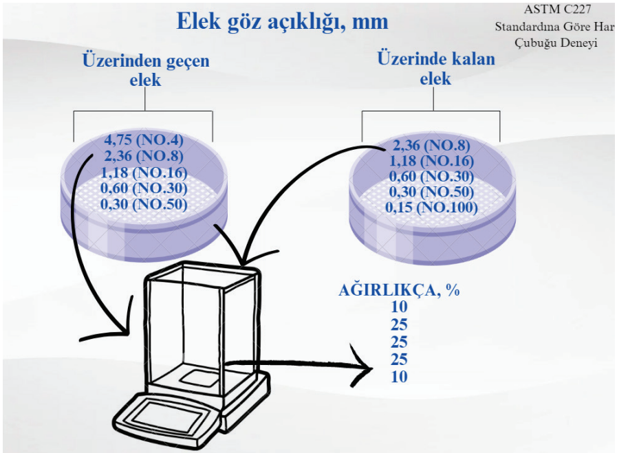
Şekil 6. Agregalar elek boyutları ve oranları
