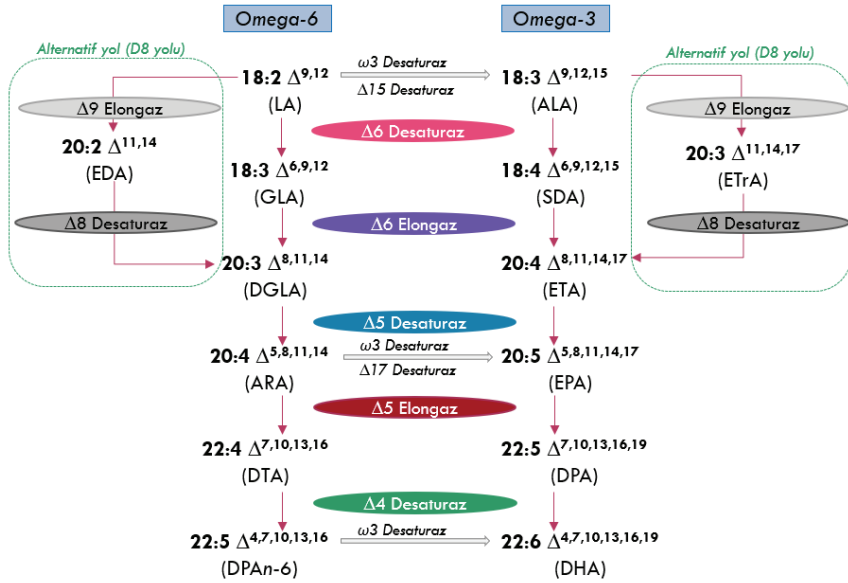
Şekil 5. Omega-3 LC-PUFA'ların biyosentezi için aerobik yolların şematik gösterimi. İlgili desaturaz, elongaz aktiviteleri ve ilişkili substratları, bazı sınırlı örneklerde gözlemlenen alternatif D8 yolu.
