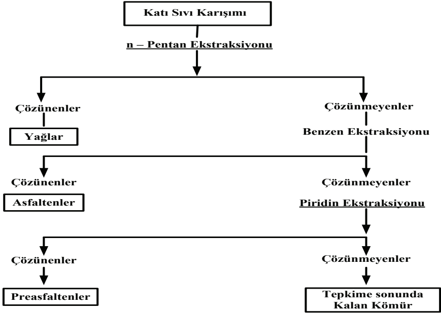
Şekil 2. Kömür Sıvılaştırma Ürünleri
