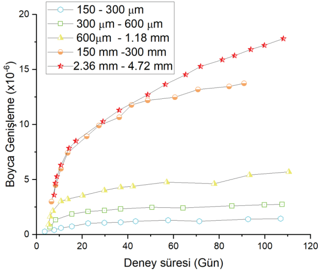
Şekil 2. Boyutları farklı reaktif agregaların boyca genleşme üzerine etkisi (Hobbs and Gutteridge, 1979.)
