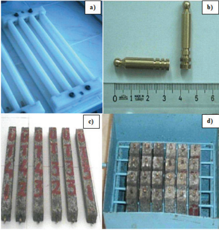
Şekil 8. ASTM C227 Standardına göre harç çubuğu deney düzeneği (a) Numune kalıplarının hazırlanması, b) numune boy ölçümlemeleri için kullanılan pimler, c) numunelerin hazırlanması, d) numunelerin ölçüm gününe kadar hazırlanan sulu çözeltide bekletilmesi)
