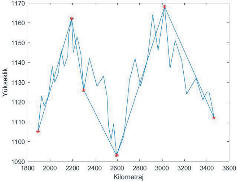
Şekil 1. Boykesit tasarımı
