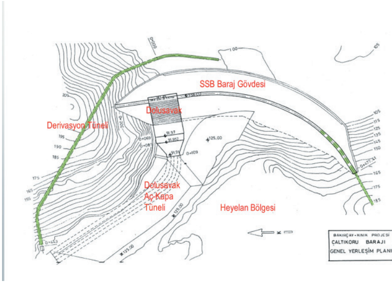
Şekil 2. Heyelandan sonra Çaltıkuru barajı genel yerleşimi.
