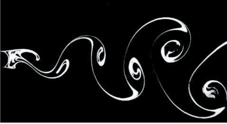
Şekil 1.1. Re=140 'ta bir silindirin arkasında bir Kármán girdap caddesi, Van Dyke'den S. Taneda'nın fotoğrafı (Van Dyke, 1988)
