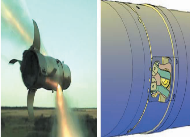
Şekil 18. Tepki Jeti Denetimli Antitank Füzesi (Živkovič vd., 2016)
