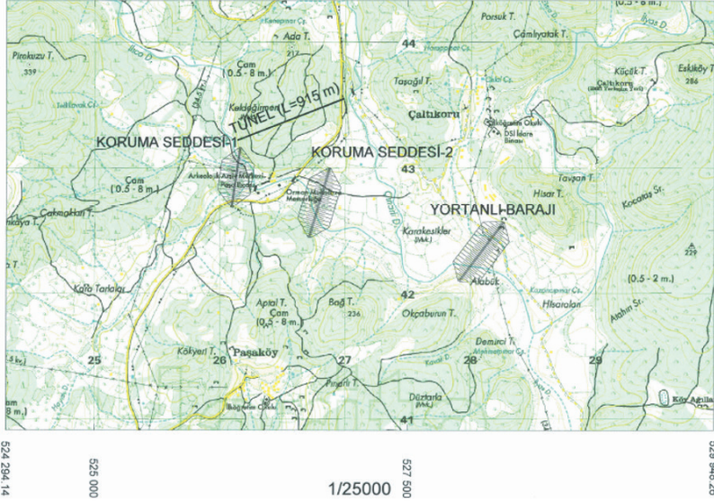
Şekil 6. Allioni Antik Kentinin Yortanlı Baraj Gölünden korunması projesi.
