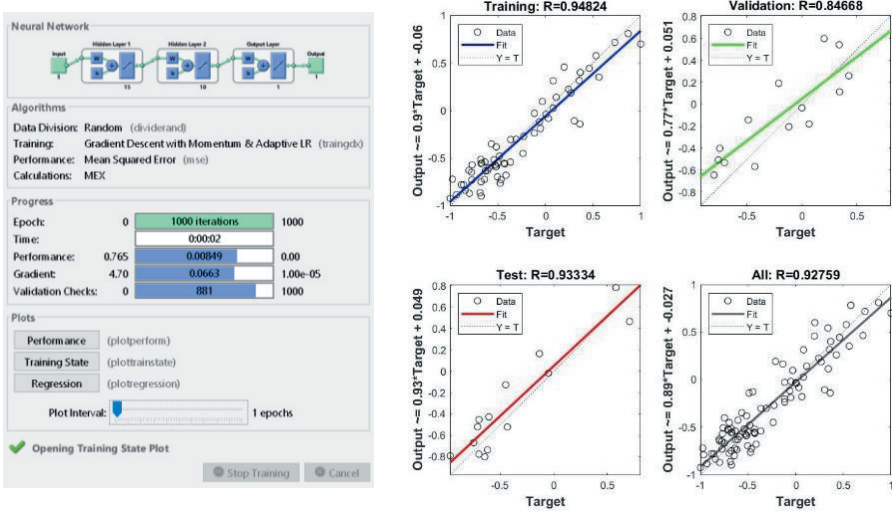
Şekil 3: Regresyon Grafikleri
