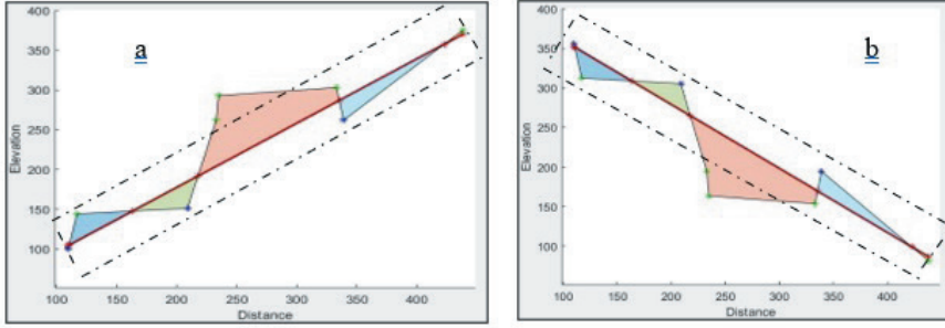
Şekil 14. Doğru parçaların ayrı ayrı optimizasyonu
