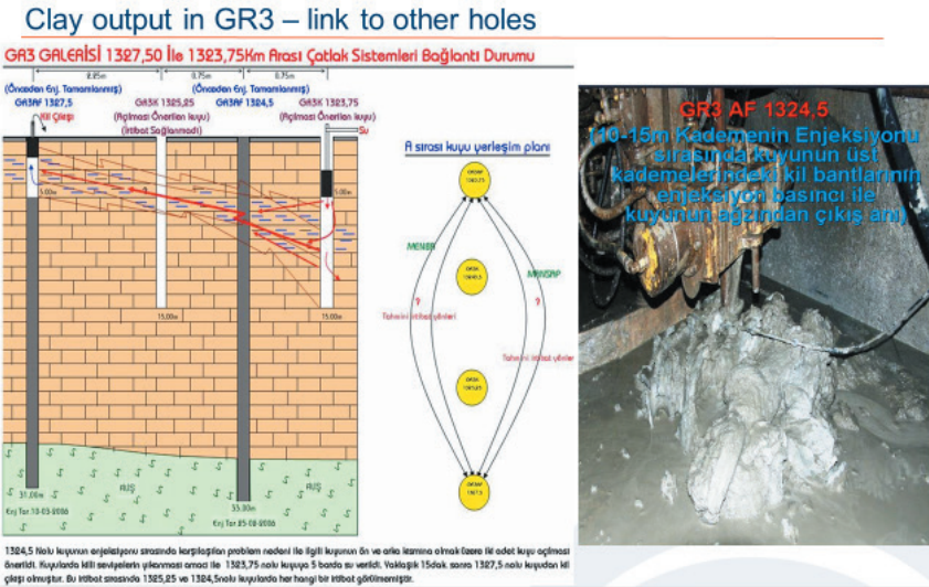
Şekil 10. Ermenek barajında çatlaklar arasında kil dolguların yıkanması için açılan kuyular (solda) kil bantlarının uygulanan 5 barlık su basınçları ile dışarı atılması (sağda) (Linortner, 2022).
