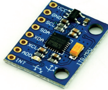
Şekil 10: MPU-6050 ivmeölçer sensörü
