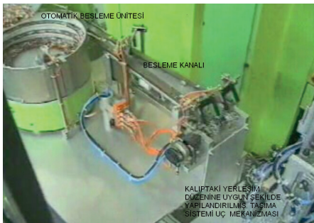
Şekil 4. Takviye Elemanı Dizgi Sistemi
