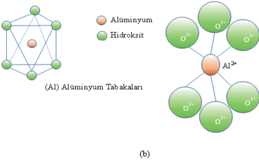
Şekil 3. (a) Silika tetrahedronu (dört yüzü silika), (b) Alümina oktahedral (sekiz yüzü alümina)
