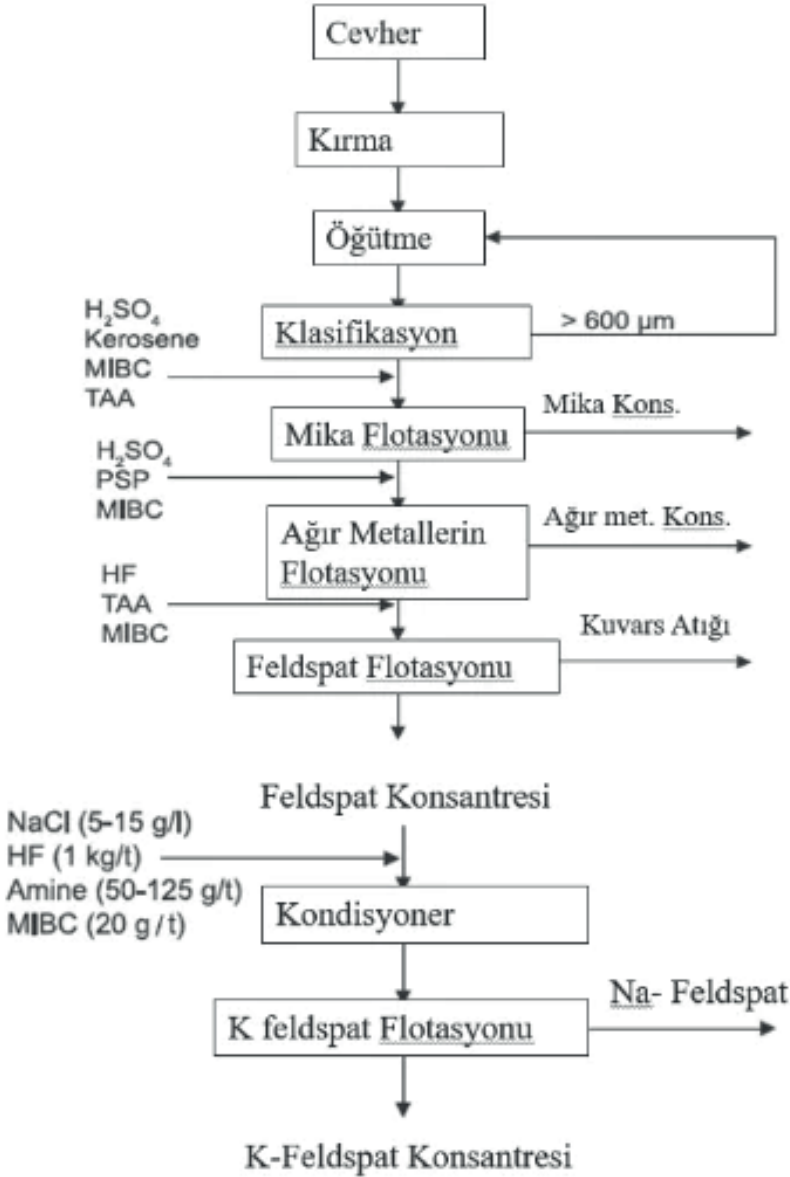
Şekil 4. Feldispatın Flotasyon Yöntemi İle Zenginleştirilmesinin Akım Şeması (URL-6).
