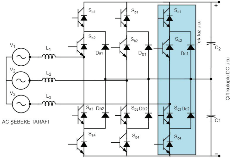
Şekil 22: Üç Fazlı Üç Seviyeli DKE Dönüştürücü (Khalid vd., 2022)
