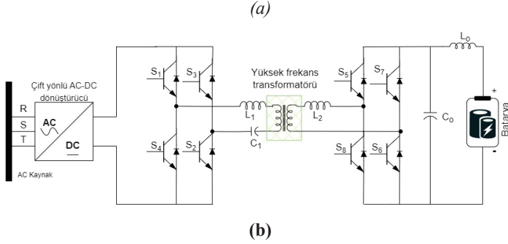
Şekil 6: (a) Çift Yönlü İzolesiz iki bölge Şarj Edici (b) Çift Yönlü İzoleli Dual Aktif Köprü Şarj Edici (Khalid vd., 2022; Yılmaz ve Krein, 2013).
