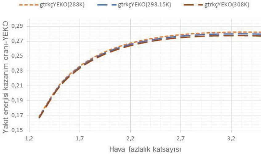
Şekil 6: Değişik kompresör giriş havası sıcaklıklarında hava fazlalık katsayısının YEKO-yakıt enerjisi kazanım oranına olan etkisinin değişimi.
