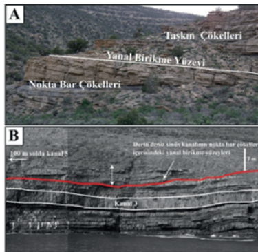
Şekil 13. (a) Menderesli akarsu sistemi içerisindeki yanal birikme yüzeyleri ve çökelleri (Reineck ve Singh, 1990); (b) Ross Formasyonu içerisindeki kumtaşı kanallarının en üst seviyesinde gelişen yanal birikme yüzeyleri ve diğer kanal elementlerinden görünüm (Wynn vd., 2007).
