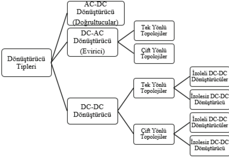
Şekil 7: Şarj Topolojisinde Kullanılan Dönüştürücü Çeşitlerinin Genel Sınıflandırması
