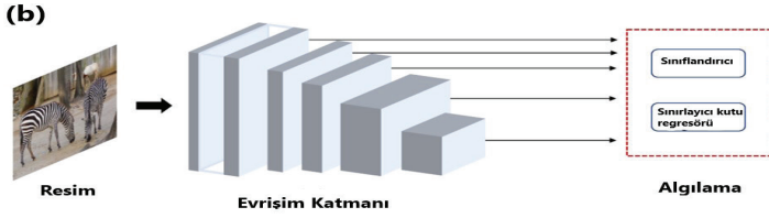
Şekil 5. SSD mimarisi
