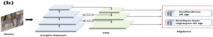
Şekil 6. RetinaNet mimarisi
