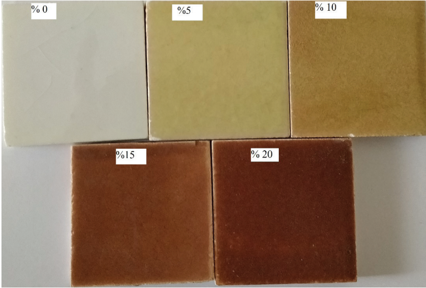
Şekil 2. Nikel cevher atıklarının kurşunlu çini sırtı içerisine ağırlıkça, % 0, %5, % 10, % 15 ve % 20 oranında ilavesi
