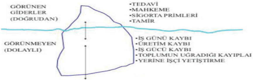
Şekil 2. Buzdağı teorisi [5]
