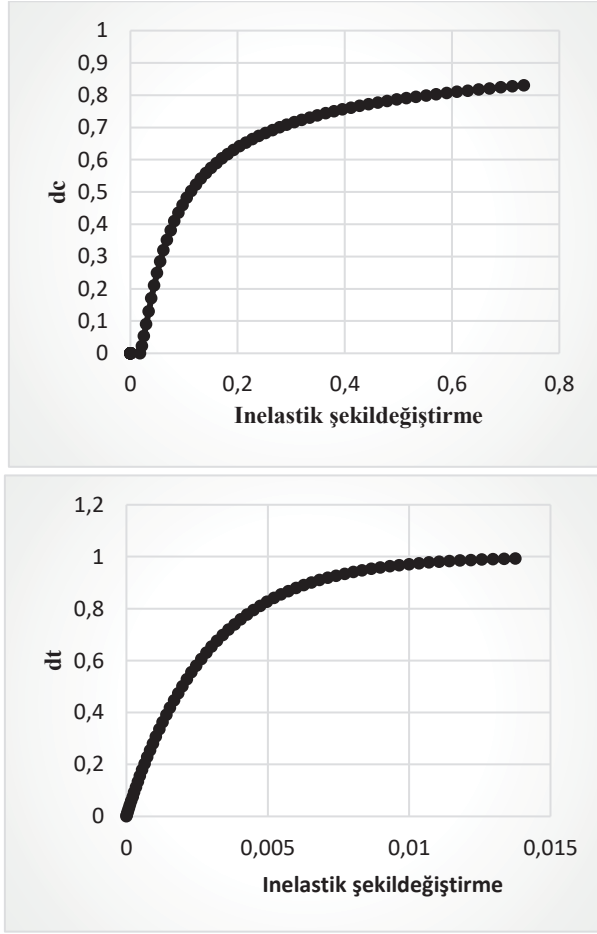
Şekil 4. Sonlu eleman modelinde kullanılan hasar parametreleri
