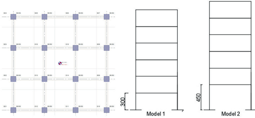
Şekil 3. Çalışmada analiz edilen yapı modellerinin planı ve zemin kat yüksekliği karşılaştırması (Model 1: 3 m, Model 2: 4,5 m).
