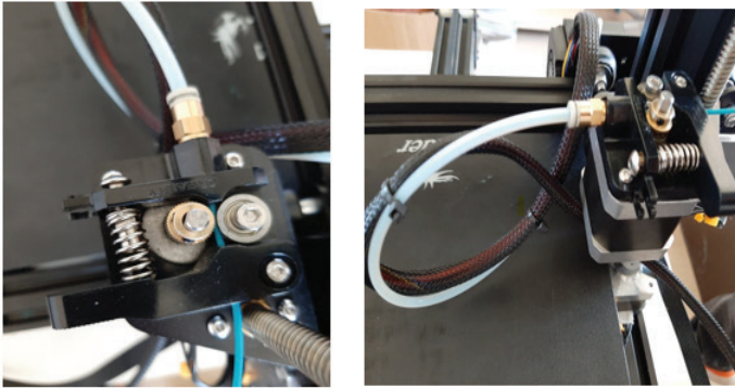
Şekil 3 Bowden Ekstrüder
