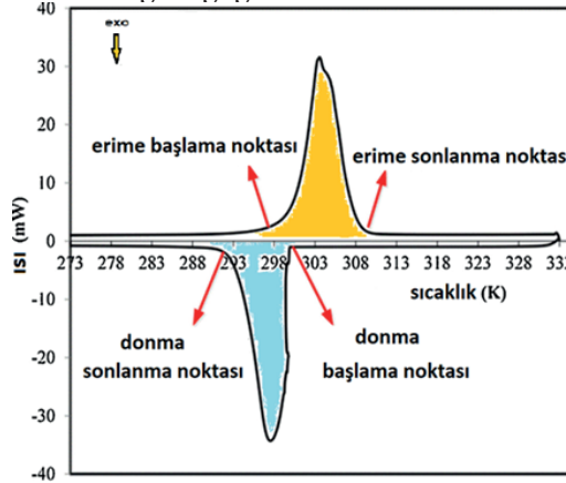
Şekil 2. FDM (n-Oktadekan) için erime ve donma süreçlerini gösteren DSC eğrileri (Kumarasamy vd., 2016).
