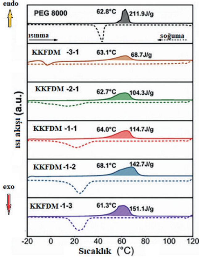
Şekil 3. PEG ve KKFDm1-3 DSC eğrisi (Zhang vd., 2025).
