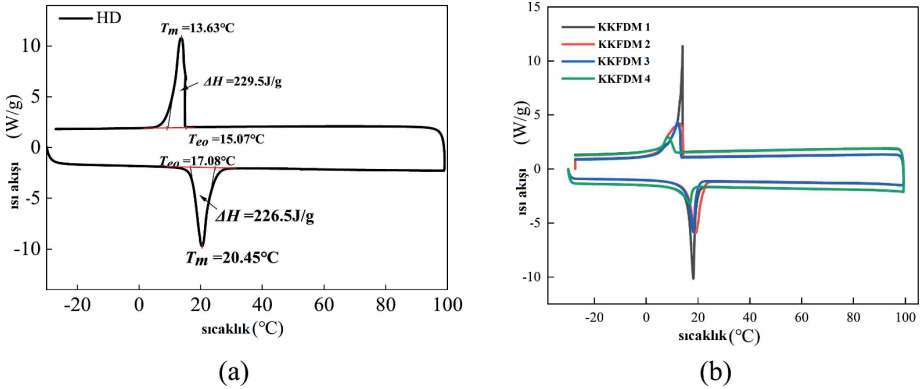
Şekil 4. DSC test sonuçları (a) n-hegzadekan (HD) ; (b) KKFDm1,2,3,4 (Wang vd.,2025).
