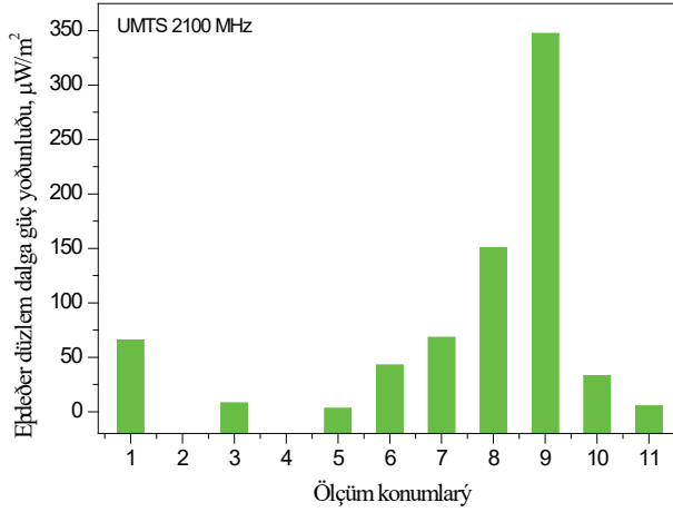
Şekil 10. UMTS 2100 MHz frekansında hesaplanan haftalık ortalama eşdeğer düzlem dalga güç yoğunluğunun ölçüm konumlarına göre değişimi
