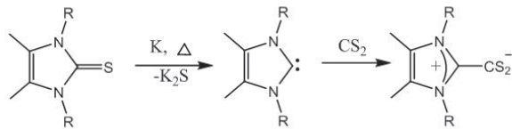
Şekil 11. Halkalı tiyoürelerden \text{NHC} \cdot \text{CS}_2 sentezi
