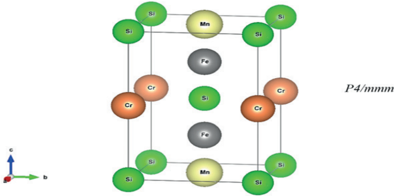
Şekil 1: \text{Fe}_2\text{Cr}_{0.5}\text{Mn}_{0.5}\text{Si} alaşımı için kristal yapı
