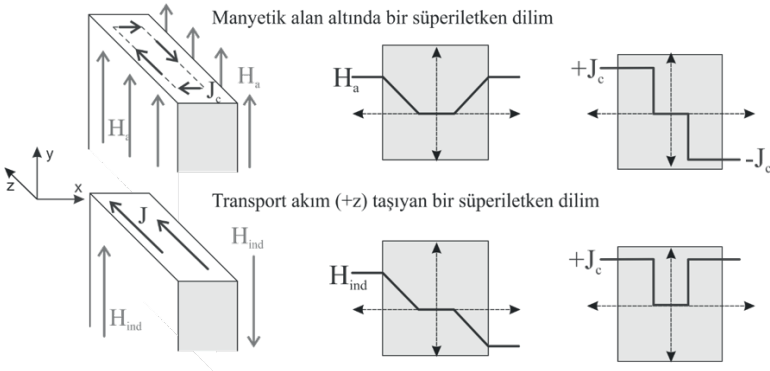
Şekil 8. (a) sadece manyetik alan ve (b) sadece transport akım uygulandığı zaman Bean Modeline göre numune içindeki alan ve akım eğrileri
