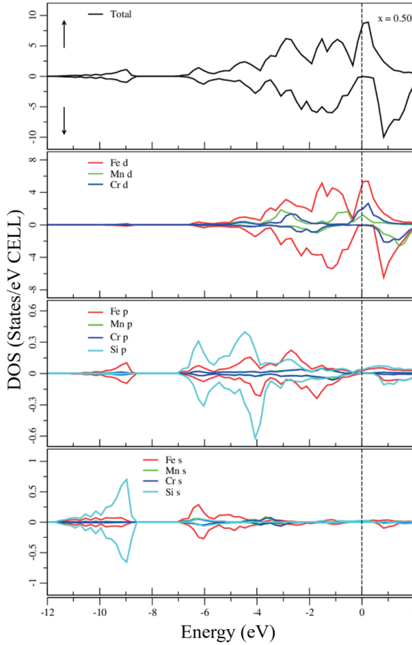
Şekil 4: \text{Fe}_2\text{Cr}_{0.5}\text{Mn}_{0.5}\text{Si} alaşımı için toplam ve kısmi durum yoğunluklar
