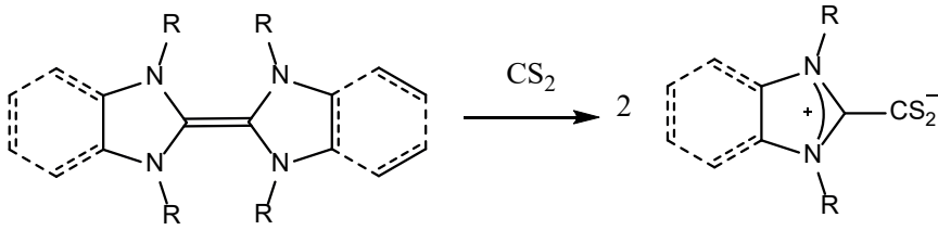
Şekil 9. Elektronca zengin entetraminlerden \text{NHC} \cdot \text{CS}_2 iç tuz sentezi
