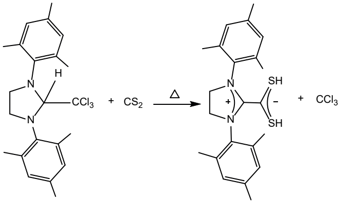
Şekil 10. Kararlı NHC öncüllerinden \text{CHCl}_3 ve \text{CS}_2 yer değiştirme tepkimesiyle \text{NHC} \cdot \text{CS}_2 sentezi
