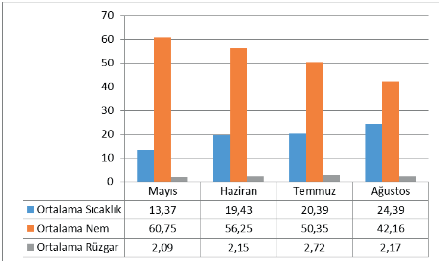
Şekil 2. Ürgüp İlçesi 2022 Yılı Meteorolojik Veriler
