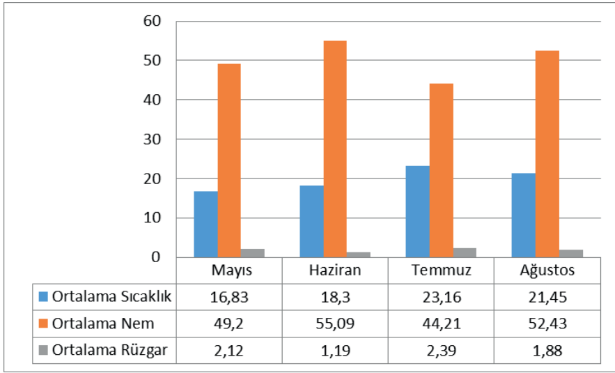
Şekil 1. Ürgüp İlçesi 2021 Yılı Meteorolojik Veriler
