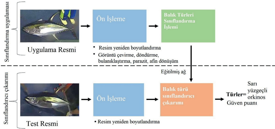
Şekil 2. Balık türlerinin sınıflandırılması için eğitim ve çıkarım hattı (Sağb ve ark., 2024)
