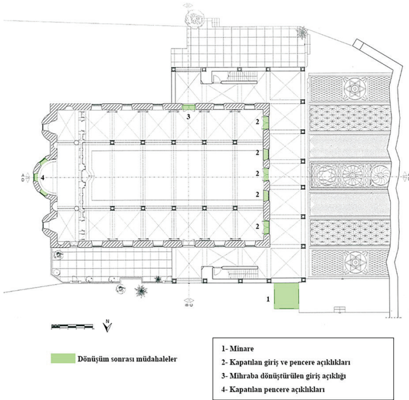
Çizim 1: Alaçatı Pazaryeri Camii Zemin Kat Planı Üzerinde Müdahale Analizi (Kaynak: Umart Mimarlık, Proje Müellifi: Salih Seymen Mimarlık)
