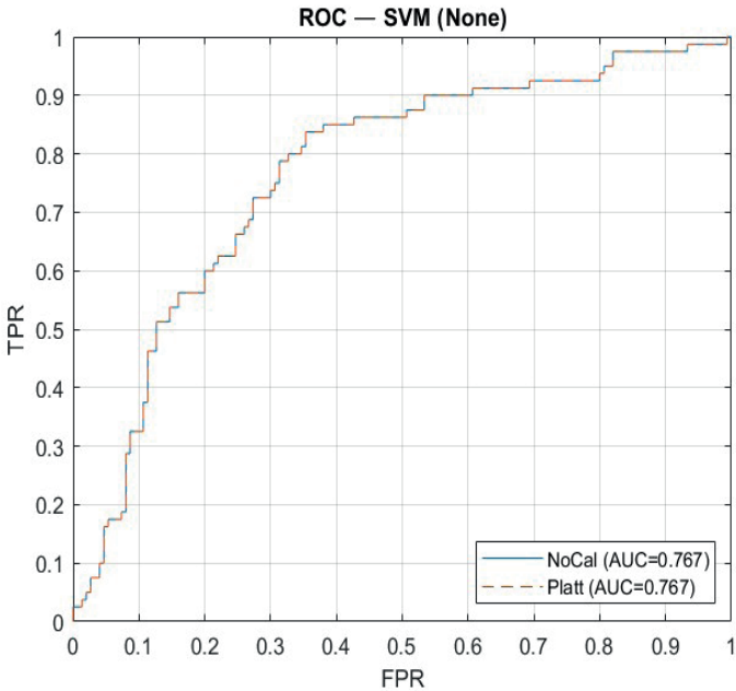
Şekil 3. SVM ROC eğrisi (ZScore yapılmadan)
