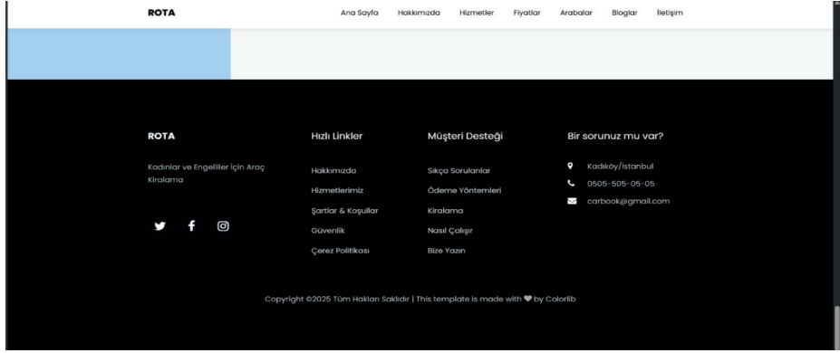
Şekil 5: Footer Bölümü
